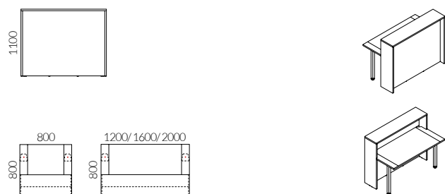
Gerade Empfangstheke hoch H:1100 mm
