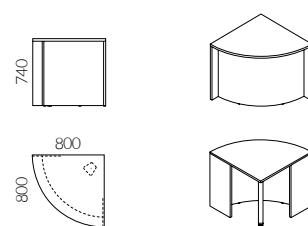
Eckelement, gebogen niedrig H:740 mm
