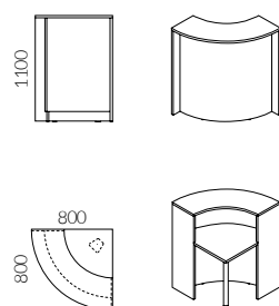
Eckelement, gebogen, hoch H:1100 mm
